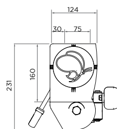
Loggia - Pose PLAFOND Sortie treuil à l'arrière
