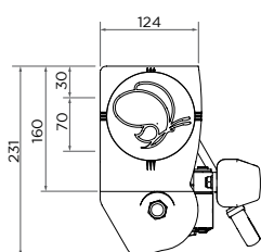
Loggia - Pose FACE Sortie treuil à l'avant (uniquement)
