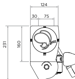
Loggia - Pose PLAFOND Sortie treuil à l'avant
